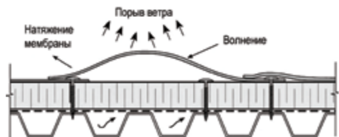
Рис. 1.1.1.1 Виды воздействий на кровлю без балласта
