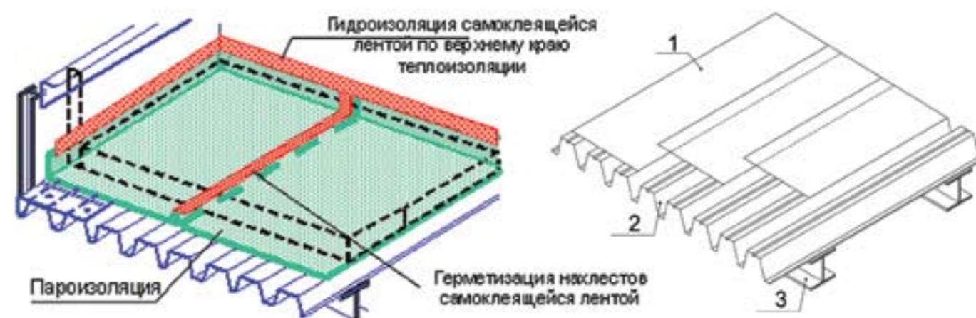
1 – пароизоляция; 2 – несущее основание (профлист); 3 – несущая конструкция. Рисунок 2.1.2 Правильная склейка нахлестов пароизоляции в системе с основанием из профлиста.
