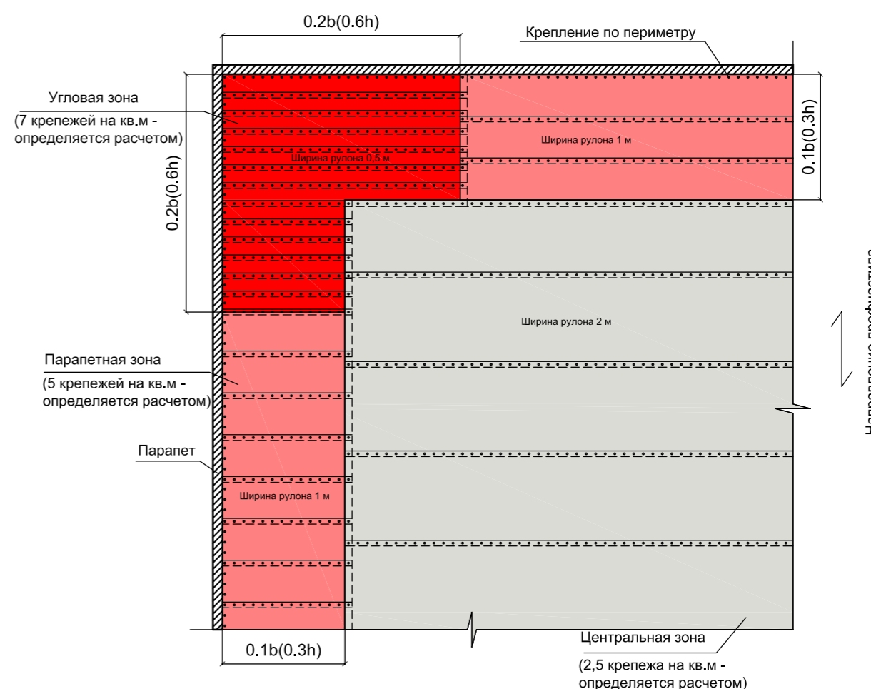
Рисунок 2.5.12. Вариант раскладки и крепления полотнищ.
