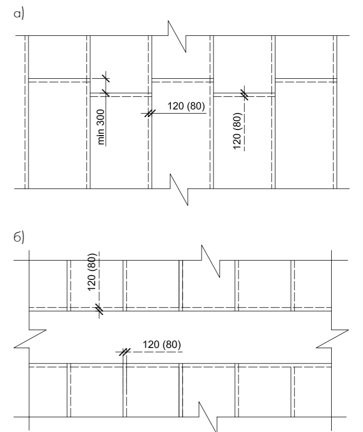
Рисунок 4.4.2 Возможные варианты расположения рулонов мембраны.
