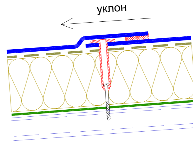
Рис. 2.4.3. "Встречный" шов.
