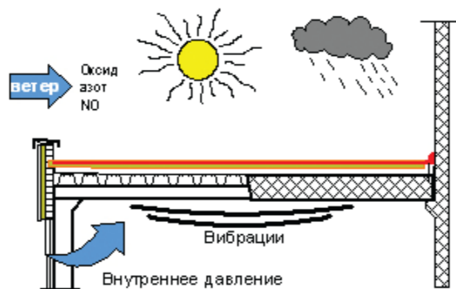
Рис. 1.1.1.1 Виды воздействий на кровлю без балласта
