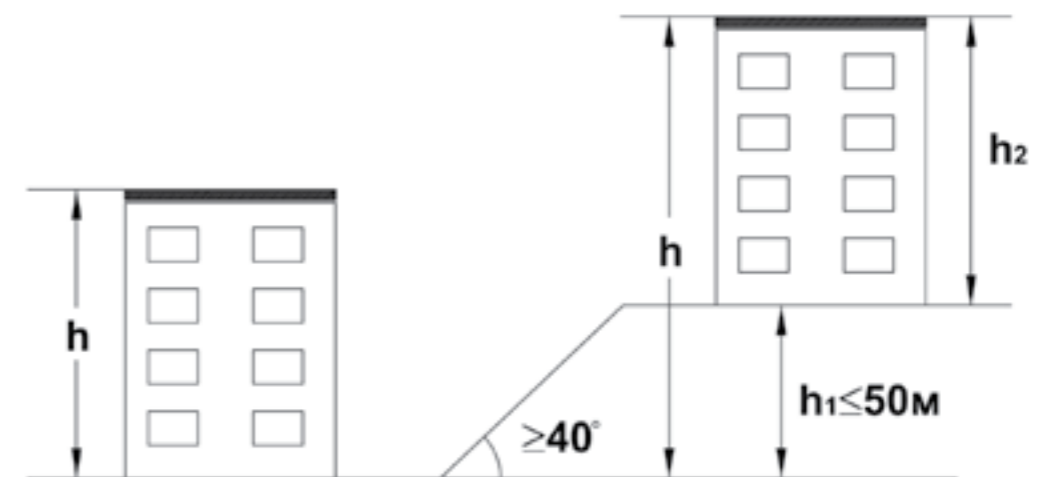
Рисунок 2.5.2. К определению высоты здания.
