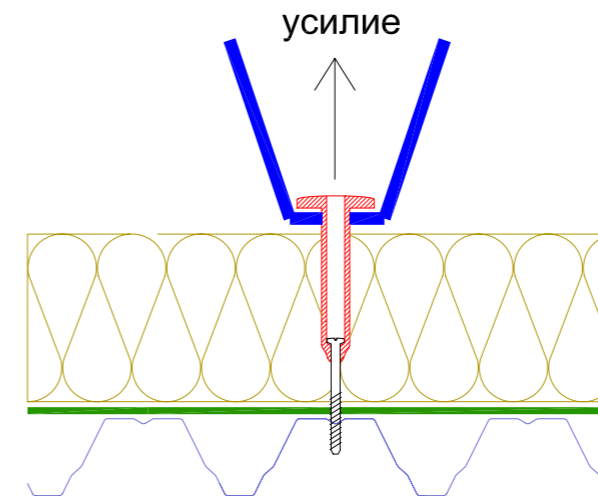
Рисунок 2.5.6 Визуальный метод определения надежности установки крепежа.
